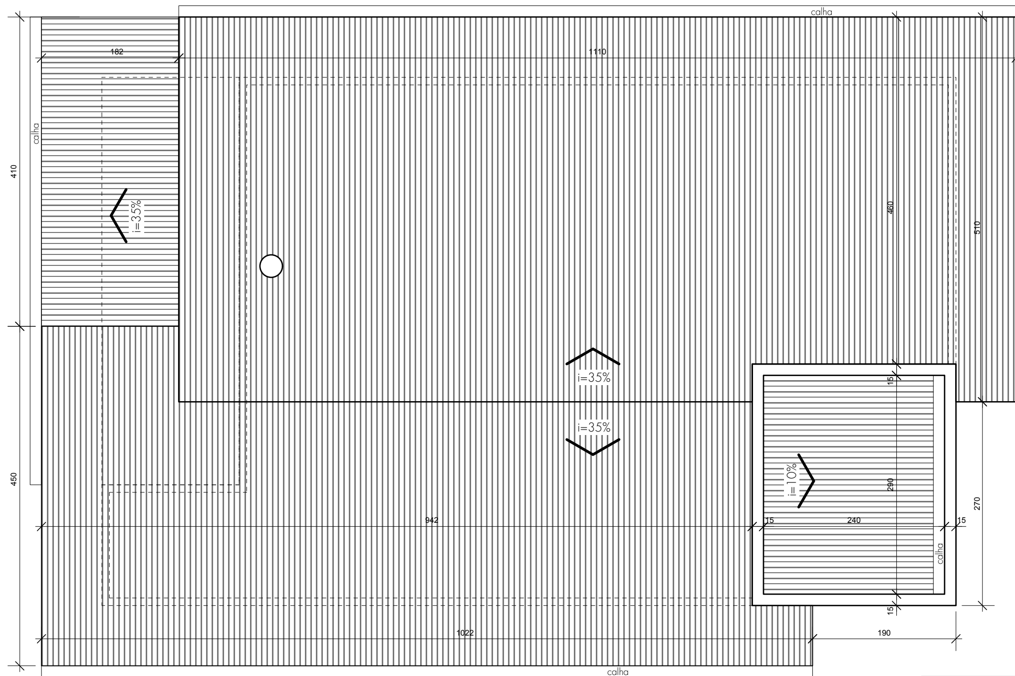
Planta de Telhado Escala: 1/50
