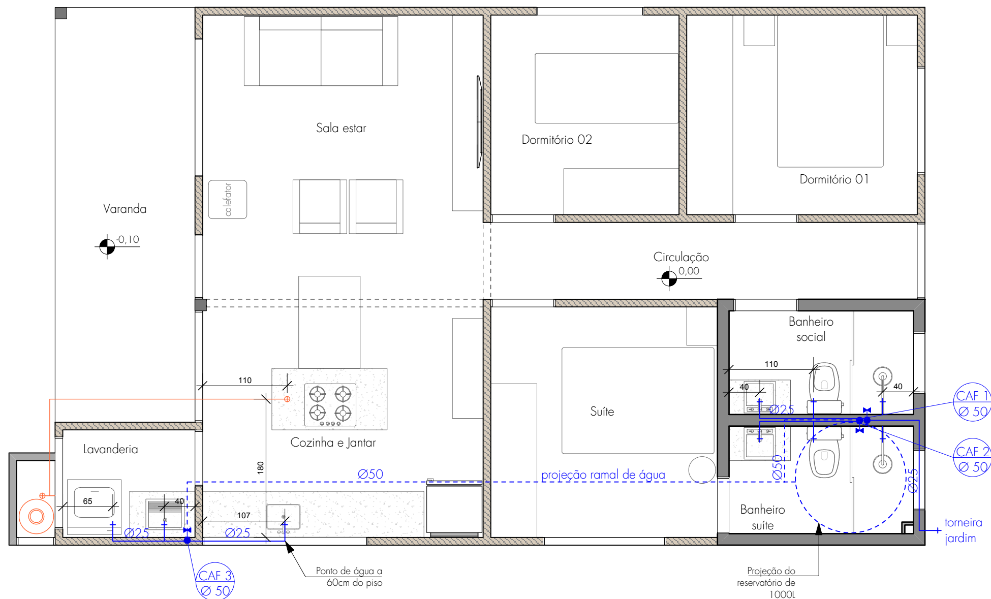
Planta Baixa Hidráulica Escala: 1/50
