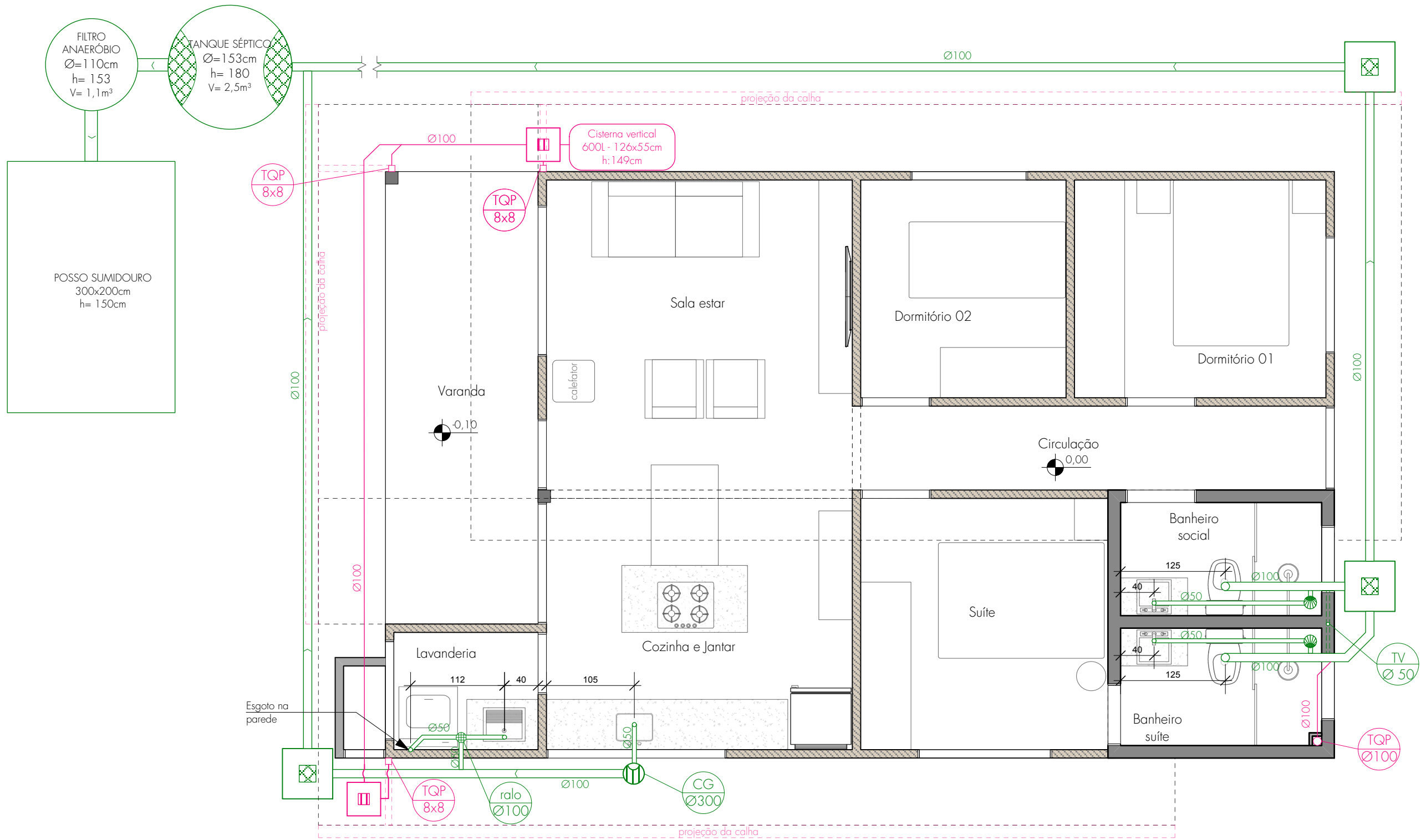
Planta Baixa Sanitário Escala: 1/50
